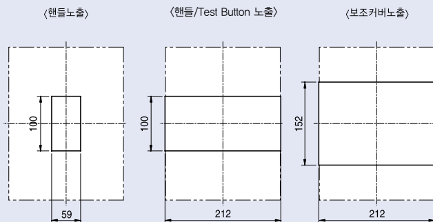
패널커버절단치수
