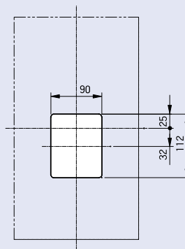
패널커버절단치수
