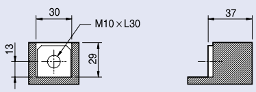
단자부 상세도
