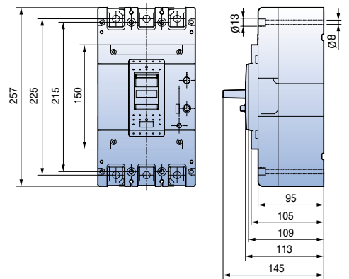
(외형도 4)
