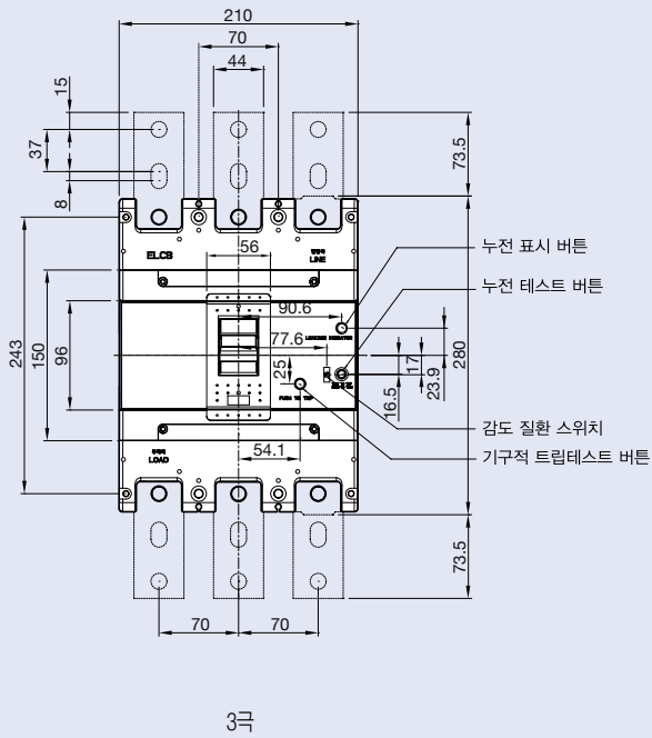
단자부 상세도
