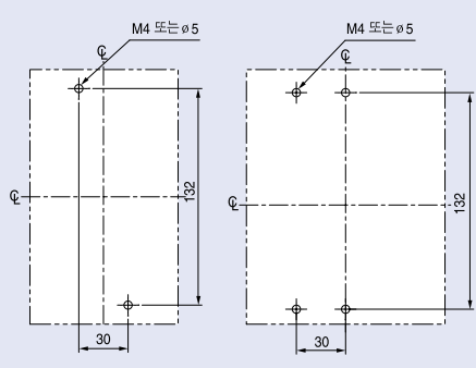
3극 4극
