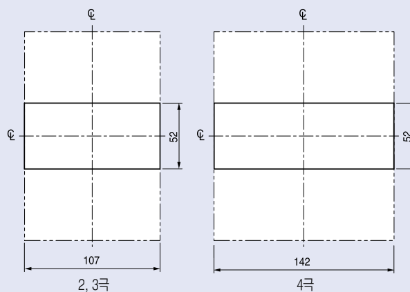
패널커버절단치수
