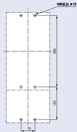
패널설치치수
