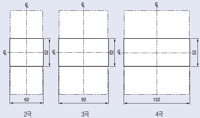
패널커버절단치수
