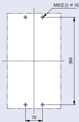
패널설치치수
