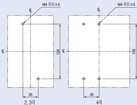
패널설치치수
