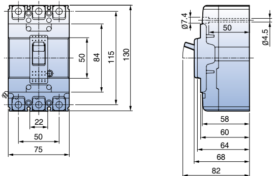
(외형도 1)
