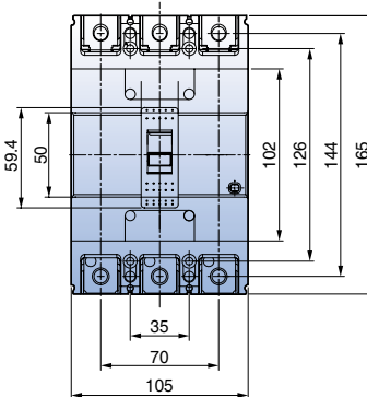
(외형도 3)
