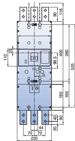
(외형도 6)
