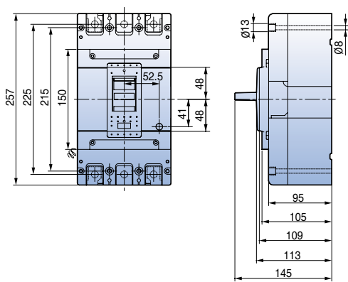
(외형도 4)
